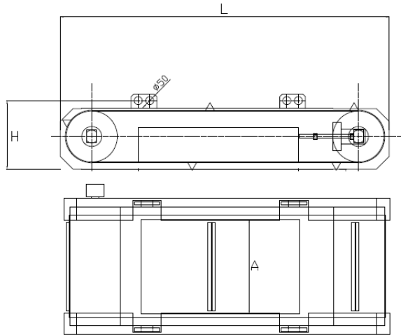
Esquema y medidas básicas de los equipos R-OMP
